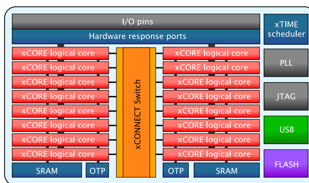
xCORE-200™ XUF216
